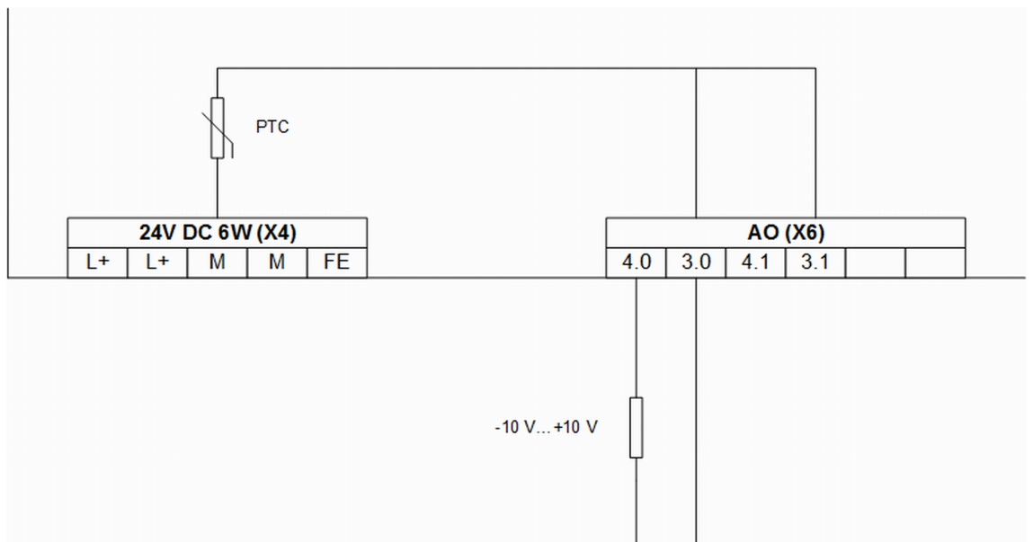
Fig. 37: Voltage output
